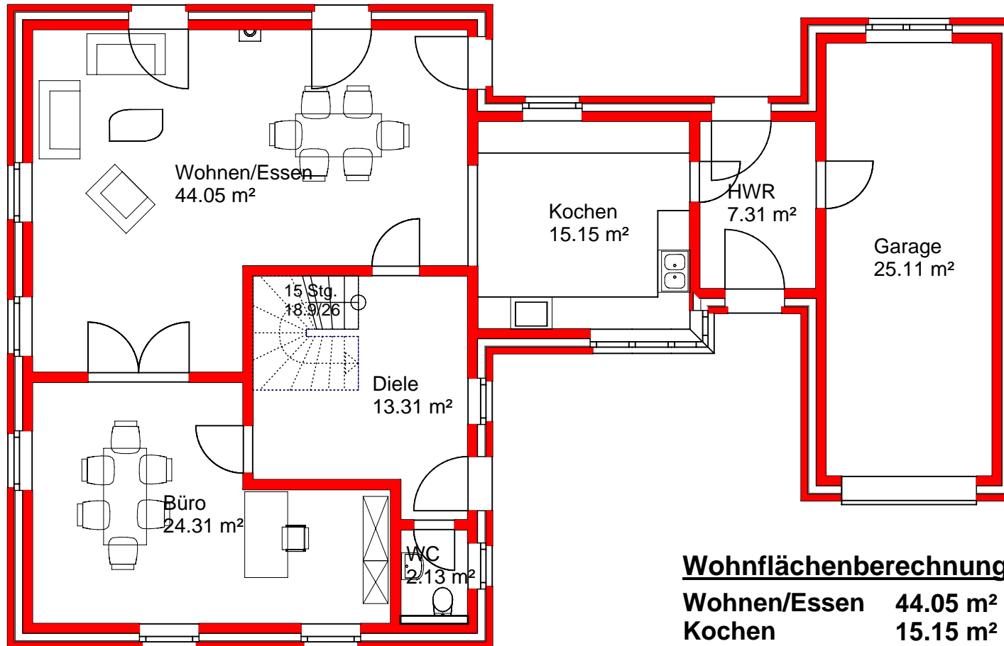
Grundriss Erdgeschoss
