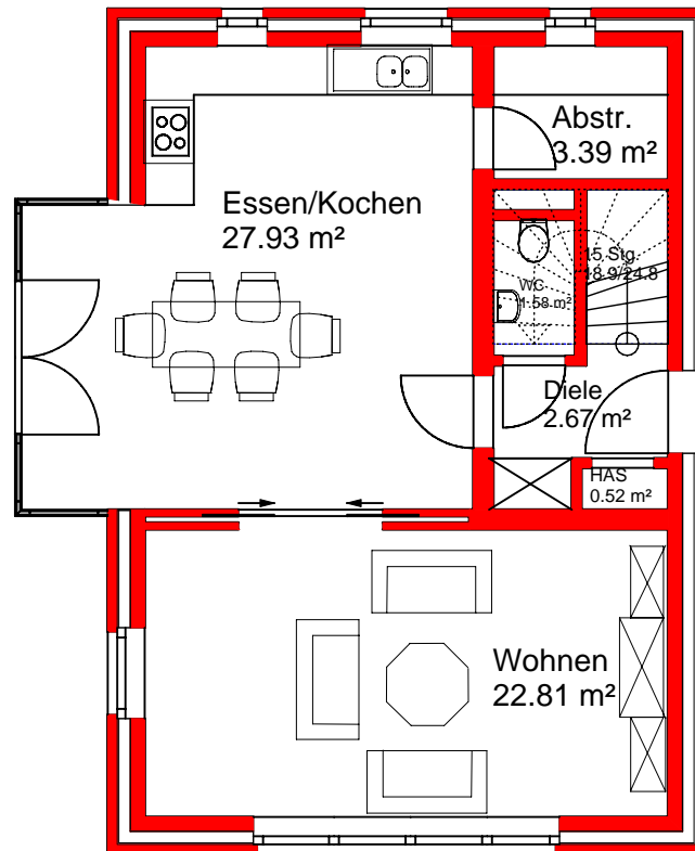
Grundriss Erdgeschoss
