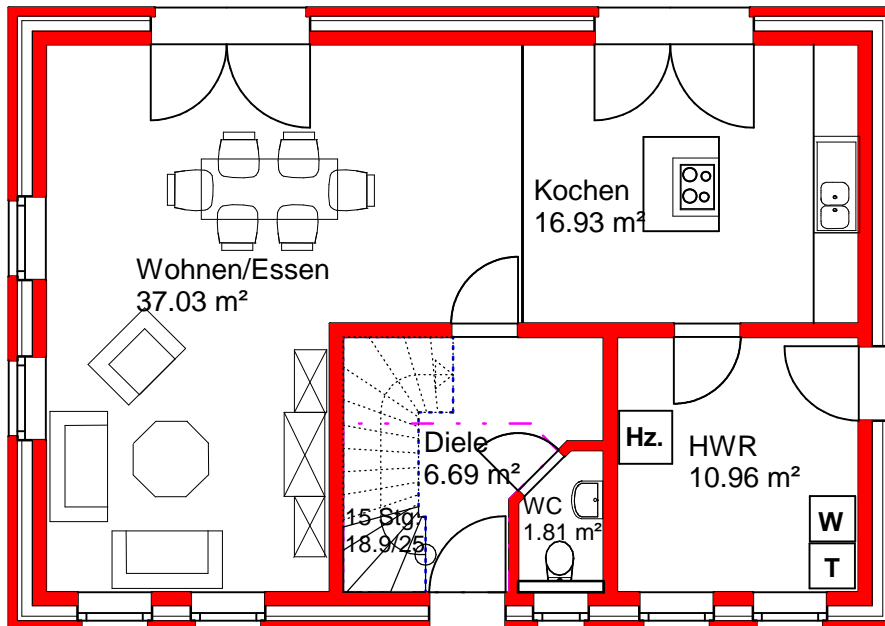
Grundriss Erdgeschoss
