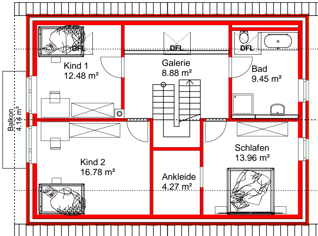
Grundriss Dachgeschoss
